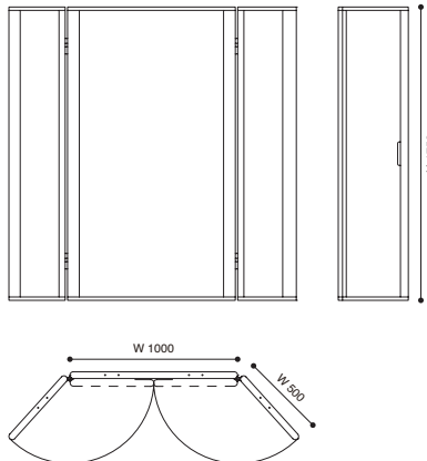
375-01/02/03 スクリーン
