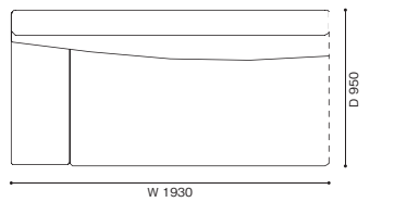
249-17 /18 2人掛エンドユニット 右/左サイドテーブル付
