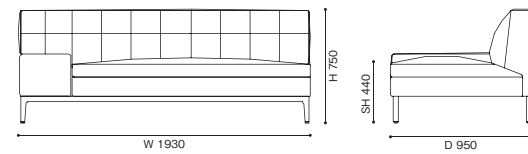
249-19 2人掛センターユニット
